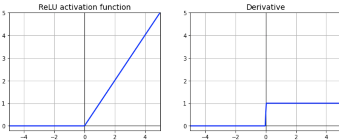
Figura 5 - Função ReLu
