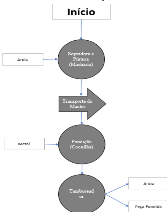
Figura 9 – Fluxo do processo futuro com a substituição do macho Hot Box para Shell
