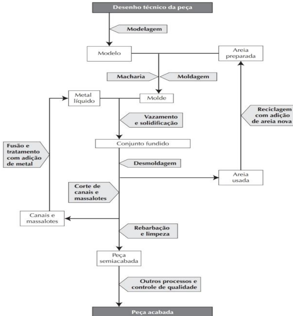
Figura 1 – Operações básicas para a produção de uma peça fundida
