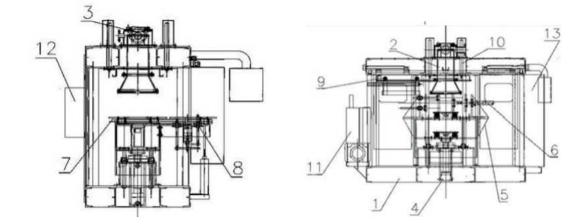
Figura 2 – Diagrama esquemático de uma sopradora de machos
