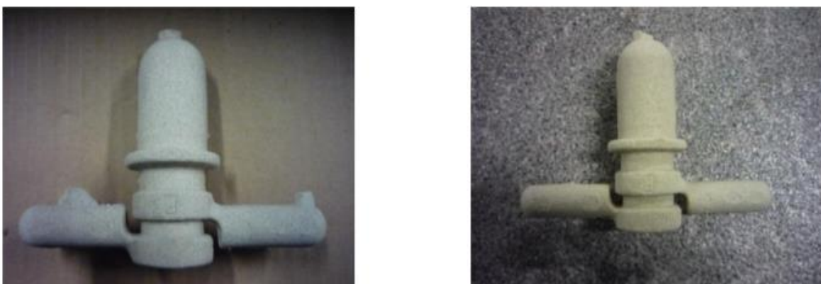
Figura 3 – Macho Hot Box antes da rebarbação (esquerda) e após rebarbação (direita)
