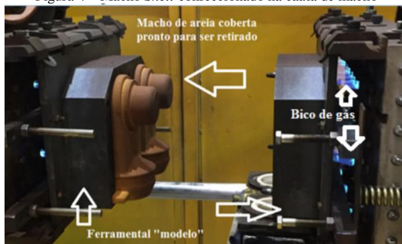
Figura 4 – Macho Shell confeccionado na caixa de macho
