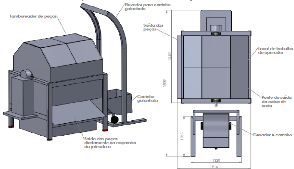
Figura 11 – Tamboreador e componentes
