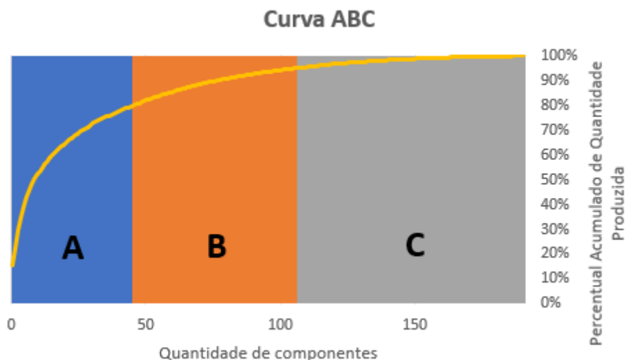
Figura 10 – Extratificação da quantidade produzida por componente na fundição estudada
