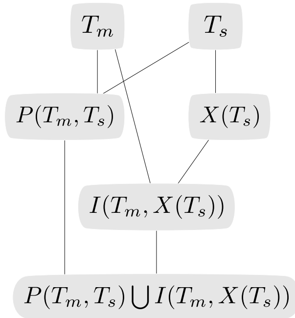
Figura 18: Diagrama representando as principais etapas do algoritmo de diferença entre templates binários, sem a utilização da operação de intersecção.
