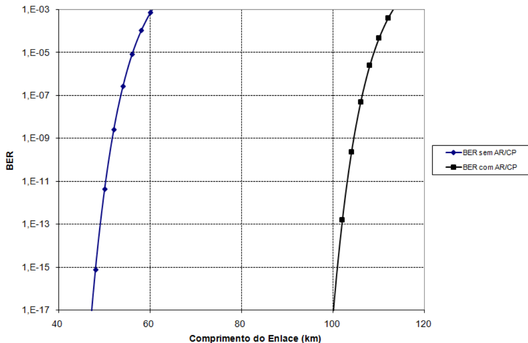
Figura 33 – Curva de BER para sistema operando em 10 Gbps. A curva em azul representa a variação da BER sem o uso do dispositivo AR/CP (teste a). A curva em preto representa a BER com o uso do dispositivo (teste c).
