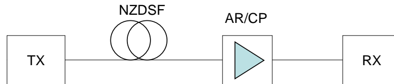
Figura 26 – Configuração simplificada do enlace óptico testado numericamente.
