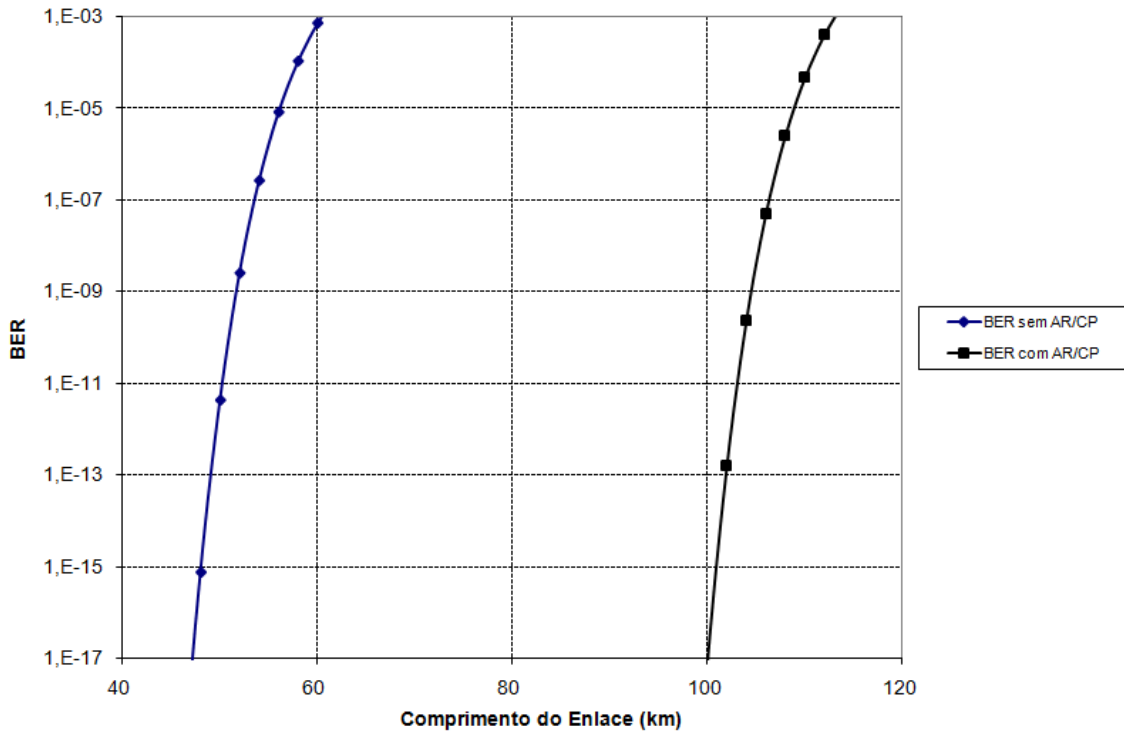
Figura 31 – Curva de BER em função do comprimento da NZDSF para sistema operando em 10 Gbps. A curva em azul representa a variação da BER sem o uso do dispositivo AR/CP. A curva em preto representa a BER com o uso do dispositivo.
